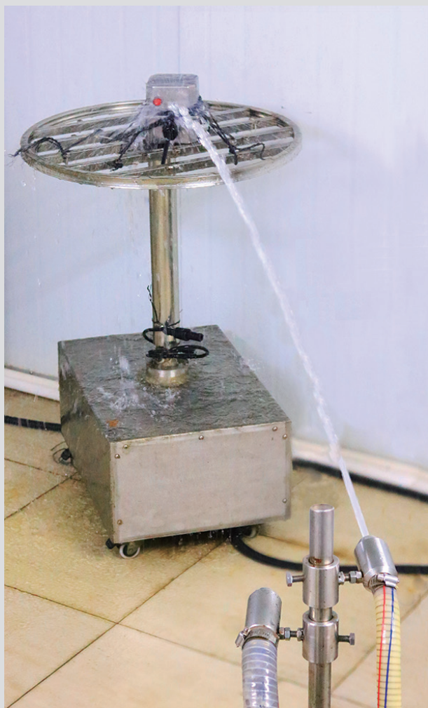
Prueba IPx5
